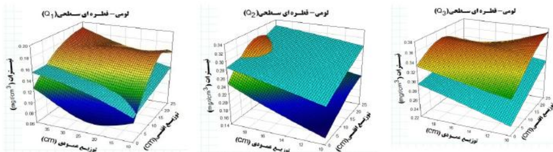
شکل ۵ مقادیر اندازه‌گیری و شبیه‌سازی شده توزیع دو بعدی نیترات در خاک لومی برای دبی‌های مورد بررسی
