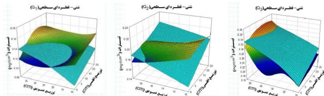
شکل ۶ مقادیر اندازه‌گیری و شبیه‌سازی شده توزیع دو بعدی نیترات در خاک شنی برای دبی‌های مورد بررسی
