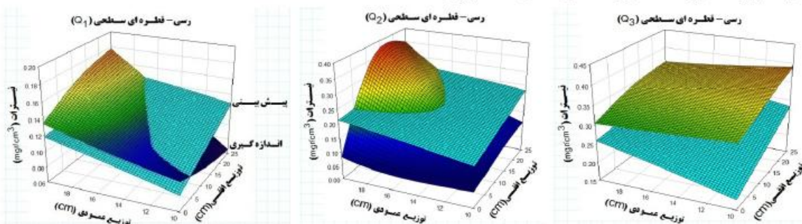
شکل ۴ مقادیر اندازه‌گیری و شبیه‌سازی شده توزیع دو بعدی نیترات در خاک رسی برای دبی‌های مورد بررسی
