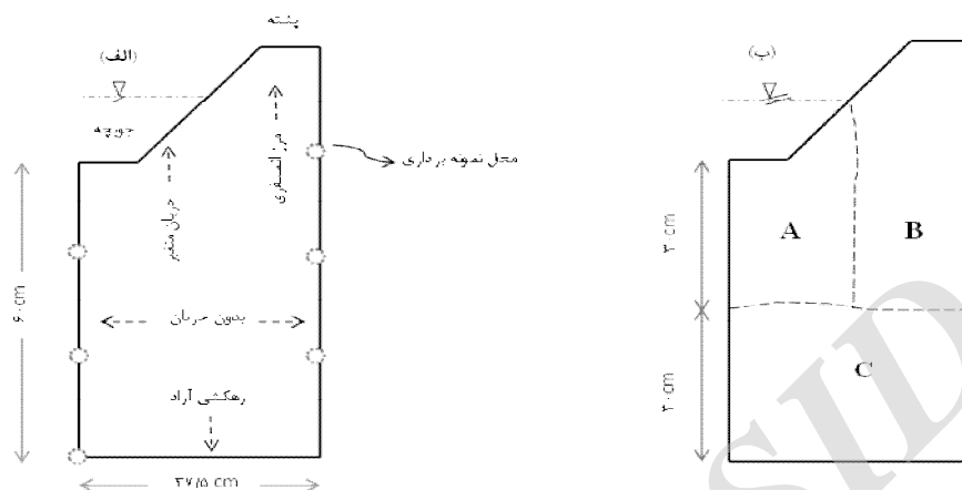
شکل ۱- الف) - شرایط مرزی اعمال شده برای جریان در مدل HYDRUS- 2D و محل نقاط نمونه‌برداری از زیر جویچه و پشته‌ها. ب) - تقسیم بندی لایه‌های خاک مورد بررسی
