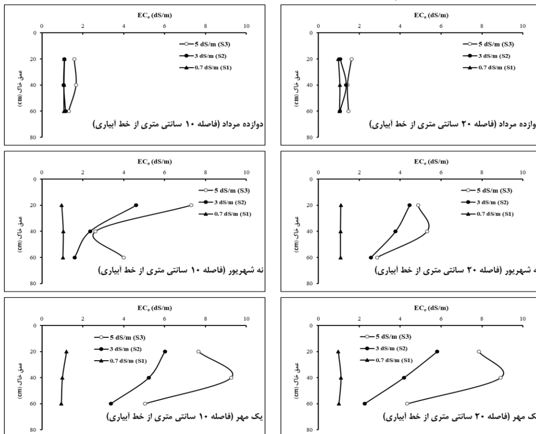
شکل ۳- نیمرخ شوری در لایه‌های ۲۰-۰، ۴۰-۲۰ و ۶۰-۴۰ سانتی‌متری و فواصل ۱۰ و ۲۰ سانتی‌متر از خط آبیاری در روزهای مختلف فصل رشد برای تیمارهای V_3S_1 ، V_3S_2 و V_3S_3
