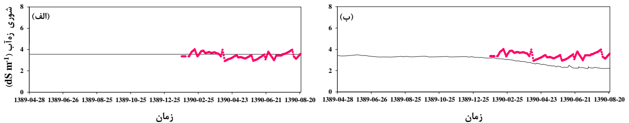
شکل ۴- مقایسه مقادیر اندازه‌گیری و شبیه‌سازی شده شور زه‌آب خروجی از سیستم زهکش زیرزمینی در شرایط اعمال (الف) و عدم اعمال (ب) فرآیند جذب سطحی املاح
