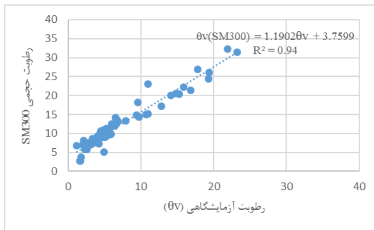
شکل ۵- رابطه بین رطوبت حجمی حس گر SM300 با رطوبت حجمی آزمایشگاهی (%)
