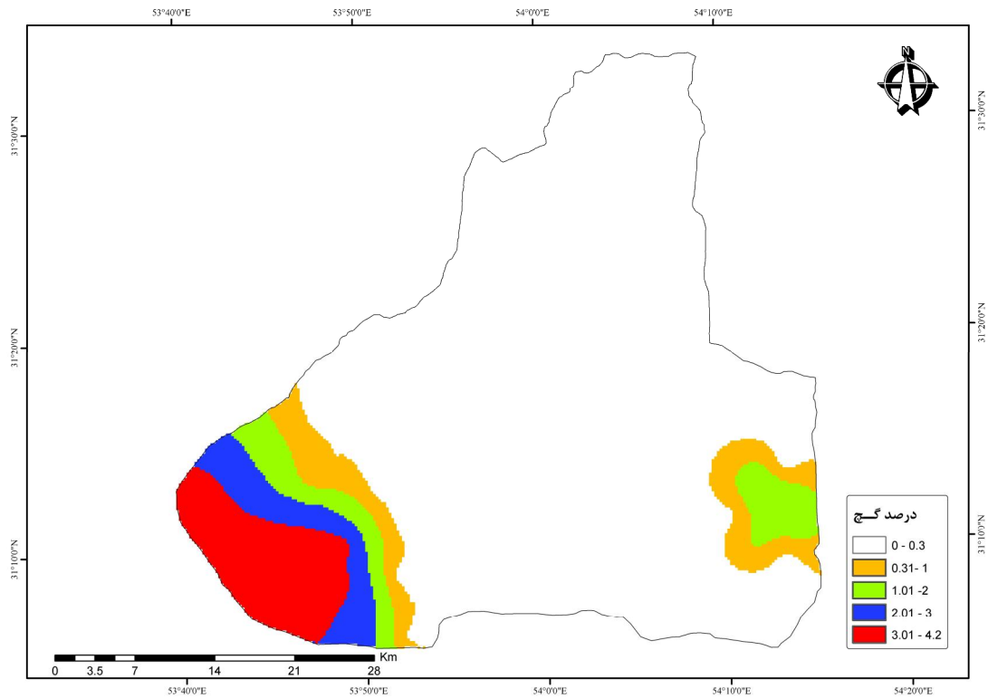
شکل ۸. نقشه درصد گچ عمق اول خاک‌های مراتع پشتکوه با استفاده از روش کریجینگ
