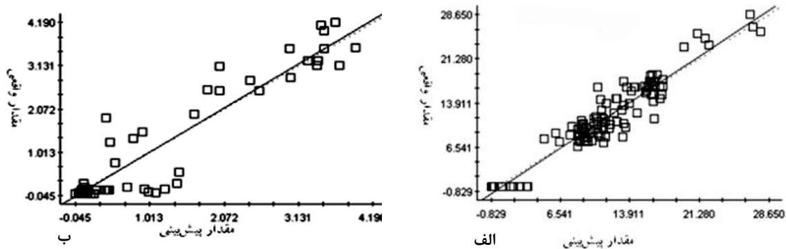
شکل ۴. ارزیابی برآورد (الف) سنگریزه عمق اول خاک و (ب) گچ مربوط به عمق اول خاک با استفاده از روش کریجینگ نقطه‌ای
