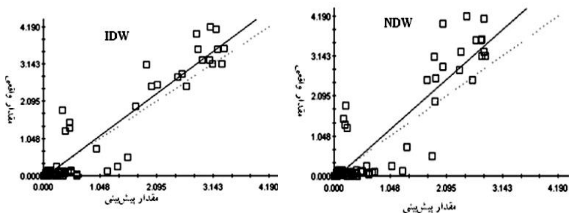
شکل ۶. ارزیابی برآورد گچ عمق اول خاک منطقه مورد مطالعه با استفاده از روش‌های وزن‌دهی نرمال فاصله (NDW) و وزن‌دهی معکوس فاصله (IDW)
