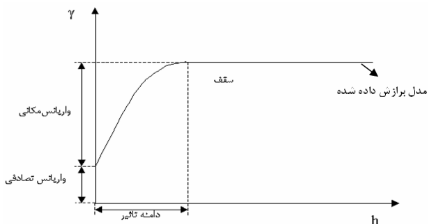
شکل ۲. نمای کلی یک واریوگرام
