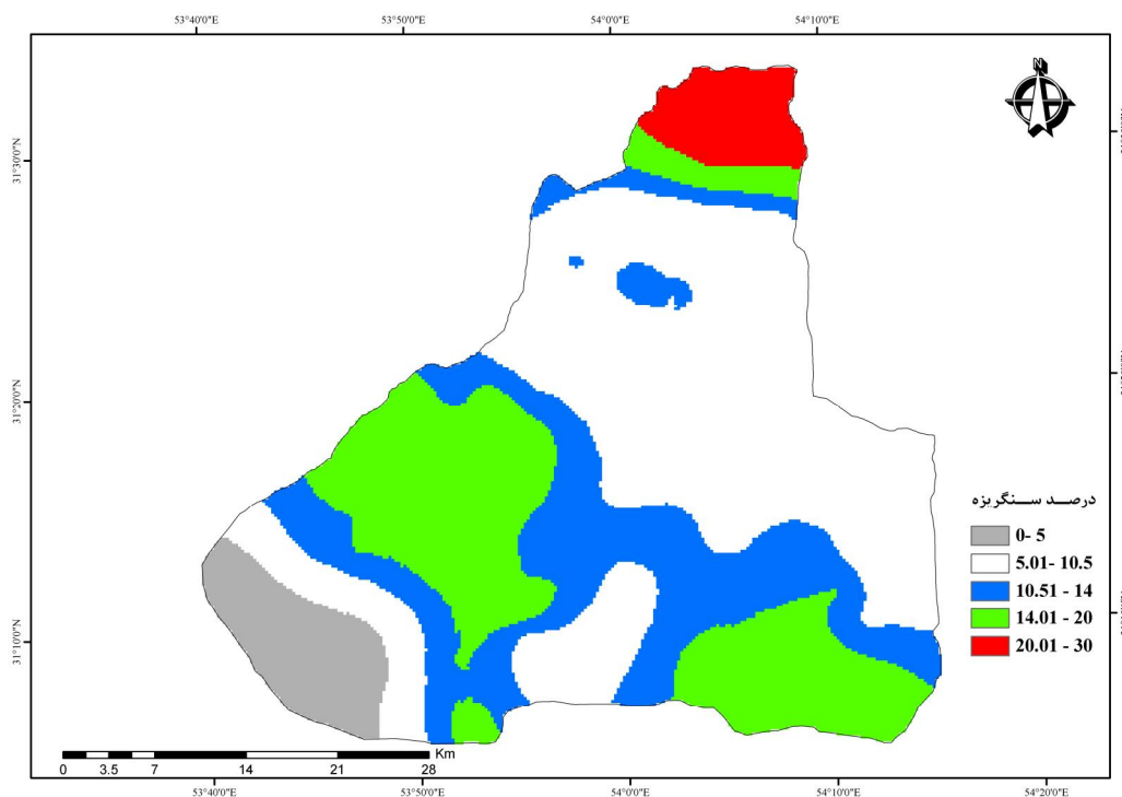
شکل ۷. نقشه درصد سنگریزه عمق اول خاک‌های مراتع پشتکوه با استفاده از روش کریجینگ
