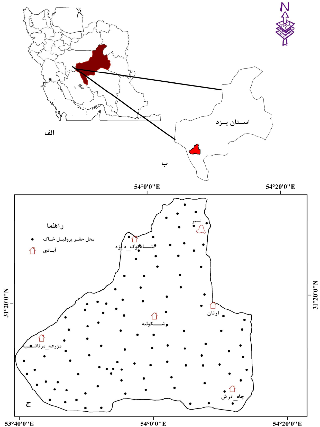
شکل ۱. موقعیت منطقه مورد مطالعه در الف) کشور، ب) استان یزد، و ج) نقشه پراکنش محل حفر پروفیل‌های خاک
