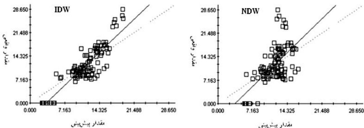
شکل ۵. ارزیابی برآورد سنگریزه عمق اول خاک منطقه مورد مطالعه با استفاده از روش‌های وزن‌دهی نرمال فاصله (NDW) و وزن‌دهی معکوس فاصله (IDW)
