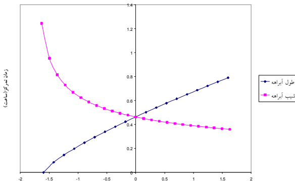
شکل ۲. نمودار آنالیز حساسیت متغیرهای رابطه کریچ
