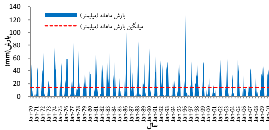
شکل ۳- نمودار بارندگی ماهانه و میانگین ایستگاه سینوپتیک بیرجند
