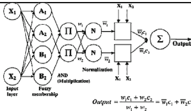
شکل ۴- شبکه [vCANFIS]
