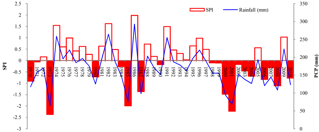
شکل ۵- انطباق خشکسالی و بارش در دوره آماری ۱۹۷۰-۲۰۱۰ ایستگاه سینوپتیک بیرجند
