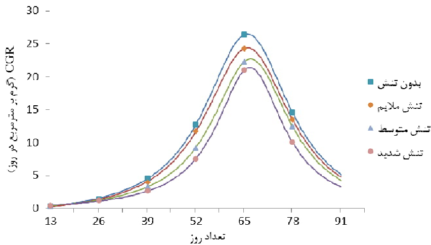
شکل ۱- رابطه بین میزان CGR (گرم بر مترمربع در روز) و تعدادروز پس از ظهورگیاه در سطح خاک تا زمان قبل از برداشت در تیمارهای مختلف تنش خشکی. خطوط منحنی نشان دهنده اعداد برازش شده (fitted) در معادلات بدون تنش، تنش ملایم، تنش متوسط و تنش شدید و علائم (بدون تنش خشکی)، (تنش ملایم)، (تنش متوسط) و (تنش شدید) میزان عددی مشاهده شده تیمارها است
