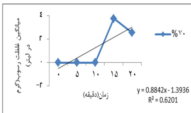
شکل ۱۴ تغییرات غلظت رسوب در طی زمان آزمایش در تیمار پوشش ۷۰٪
