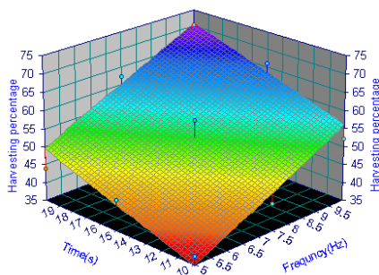
شکل ۲- تغییرات درصد برداشت بر حسب بسامد و زمان ارتعاش
