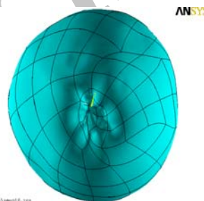
شکل ۹- مدل اجزای محدود نمونه شماره ۱۶ در نرم افزار Ansys Fig. 9. Finite element model of sample No 16 in Ansys software
