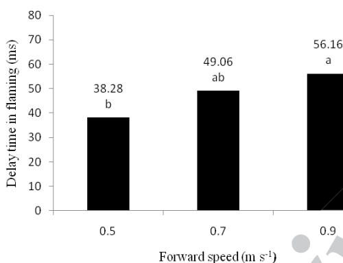
شکل ۵- مقایسه میانگین تأخیر زمانی در اعمال شعله افکنی Fig.5. Comparison of mean values of delay time in flaming
