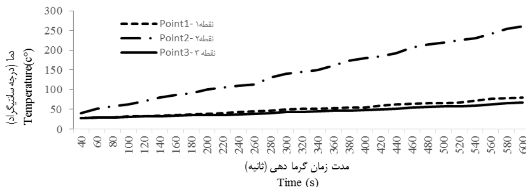
شکل ۱۲- نمودار دمای شبیه‌سازی شده- مدت زمان گرمادهی در نقاط ۱، ۲ و ۳
