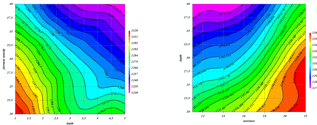
شکل 8- نمودار تغییرات جرم مخصوص ظاهری خاک با تغییر رطوبت و عمق (راست) و با تغییرات عمق و سرعت پیشروی (چپ) Fig. 8. Variation of the soil bulk density with soil moisture and depth (right) also with depth and the tractor velocity
