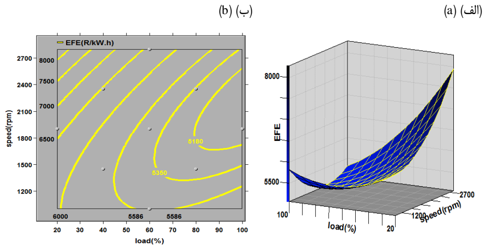
شکل ۳- نقشه رویه (شکل الف) و نقشه تراز (شکل ب) تاثیر متغیرهای بار و سرعت موتور بر روی هزینه ویژه سوخت بر حسب ریال کیلووات ساعت برای سوخت D_{62.5}B_{25}E_{12.5}
