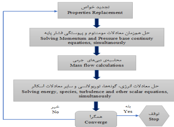
شکل ۴- روند حل مسئله در حلگر بر مبنای چگالی Fig.4. Problem solving procedure in density base solver
