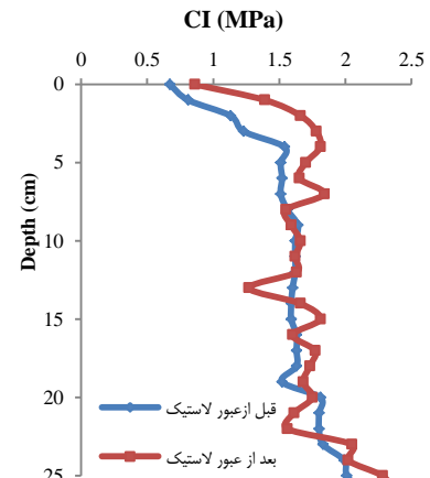
شکل ۱۶- شاخص مخروط در رطوبت ۱۴ درصد و با وزن مخصوص ۱/۴۷ گرم بر سانتی‌متر مکعب
