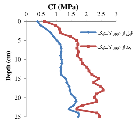
شکل ۱۵- شاخص مخروط خاک در رطوبت ۱۲ درصد با وزن مخصوص ۱/۶۹ گرم بر سانتی‌متر مکعب
