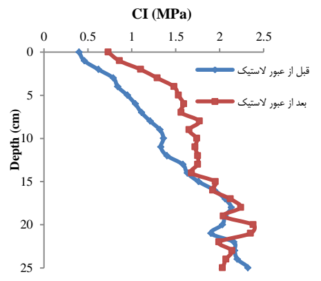
شکل ۱۲- شاخص مخروط خاک در رطوبت ۱۰ درصد با وزن مخصوص ۱/۶۹ گرم بر سانتی‌متر مکعب
