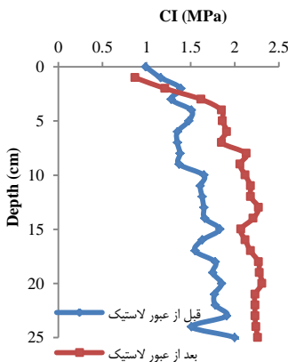
شکل ۱۱- شاخص مخروط در رطوبت ۱۰ درصد با وزن مخصوص ۱/۵۴ گرم بر سانتی‌متر مکعب
