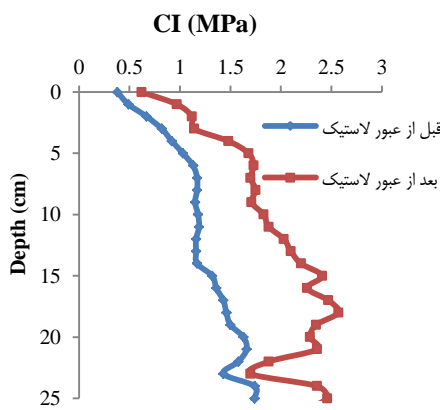
شکل ۱۴- شاخص مخروط خاک در رطوبت ۱۲ درصد و با وزن مخصوص ۱/۵۴ گرم بر سانتی‌متر مکعب
