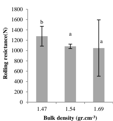
شکل ۹- مقدار میانگین مقاومت غلتشی - رطوبت ۱۴ درصد
