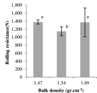
شکل ۷- مقدار میانگین مقاومت غلتشی - رطوبت ۱۰ درصد
