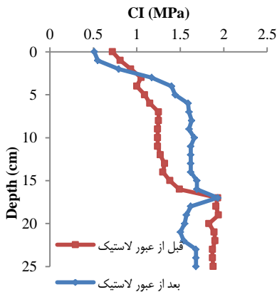
شکل ۱۳- شاخص مخروط خاک در رطوبت ۱۲ درصد و با وزن مخصوص ۱/۴۷ گرم بر سانتی‌متر مکعب
