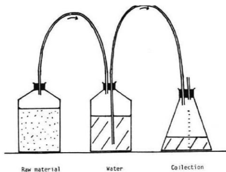
شکل ۲- روش‌های متداول اندازه‌گیری گاز خروجی از هاضم آزمایشگاهی (Raposo et al. , 2008)
