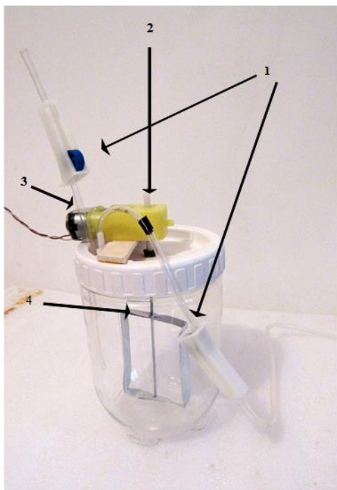
شکل ۱- نمونه هاضم مورد استفاده
