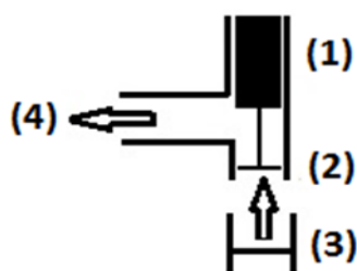
شکل ۳- ماشین پستی برقی اصلاح شده جهت برداشت گلبرگ (الف)، واحد برش اولیه (ب) و طرح‌واره‌ای از مکانیزم برش طراحی شده شامل آرمیچر (۱)، تیغه دوار (۲)، تیغه ثابت (۳) و لوله مکش (۴)
