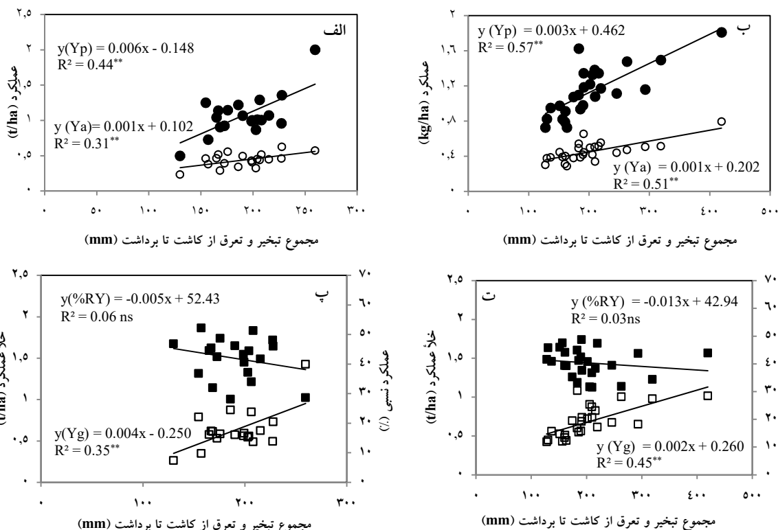
شکل ۵. رابطه بین میانگین عملکرد واقعی (Ya, ○) و پتانسیل (Yp, ●) با مجموع تبخیر و تعرق در طول فصل رشد نخود (الف) و عدس (ب) و رابطه بین خلأ عملکرد (Yg, □) و عملکرد نسبی (RY, ■) با مجموع تبخیر و تعرق در طول فصل رشد نخود (پ) و عدس (ت) در طول دوره ۱۳۸۰ تا ۱۳۹۴.
