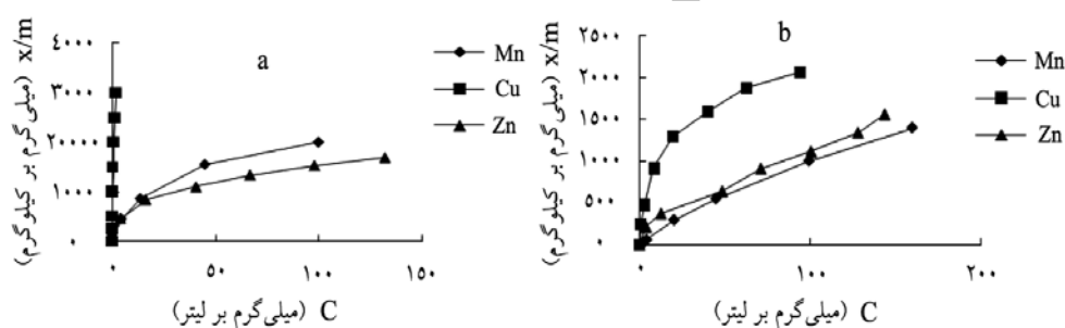
شکل ۲- منحنی‌های جذب فلزات در خاک‌های غیراسیدی و اسیدی C: میانگین غلظت تعادلی فلز، X/M: میانگین مقدار جذب شده فلز، a: خاک غیراسیدی و b: خاک اسیدی.
