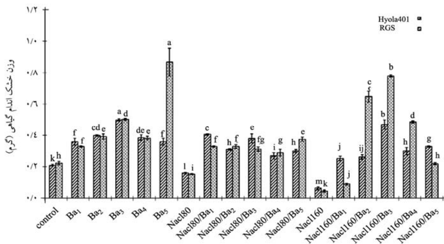
شکل ۱- وزن خشک اندام هوایی (سه گونه باکتری آزو سپریلوم: Ba_1=A. irakense DSM 11586 و Ba_2=A. irakense 49 و Ba_3=Azospirillum lipoferum 45 و دو گونه باکتری سودوموناس: Ba_4=P. fluorescens و Ba_5=P. putida )
