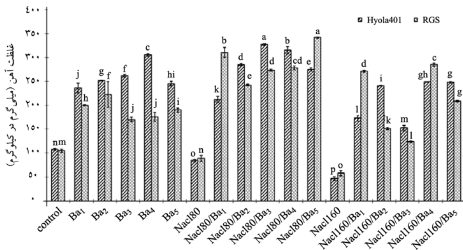
شکل ۲- میزان آهن برگ (سه گونه باکتری آروسپیریلوم: Ba_1=A. irakense DSM 11586، Ba_2=A. irakense 49 و Ba_3=Azospirillum lipoferum 45 و دو گونه باکتری سودوموناس: Ba_4=P. fluorescens و Ba_5=P. putida )
