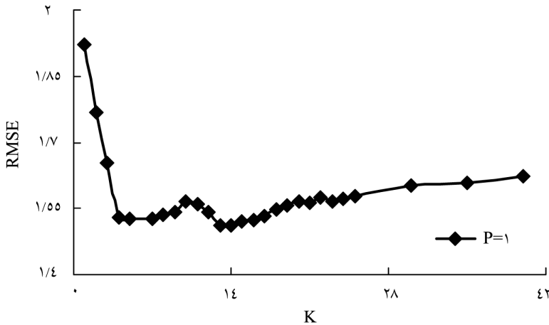
شکل ۲- تغییرات ریشه میانگین مربعات خطای برآورد CEC در تعداد مختلف نزدیک‌ترین خاک‌های همسایه (K) در P=1
