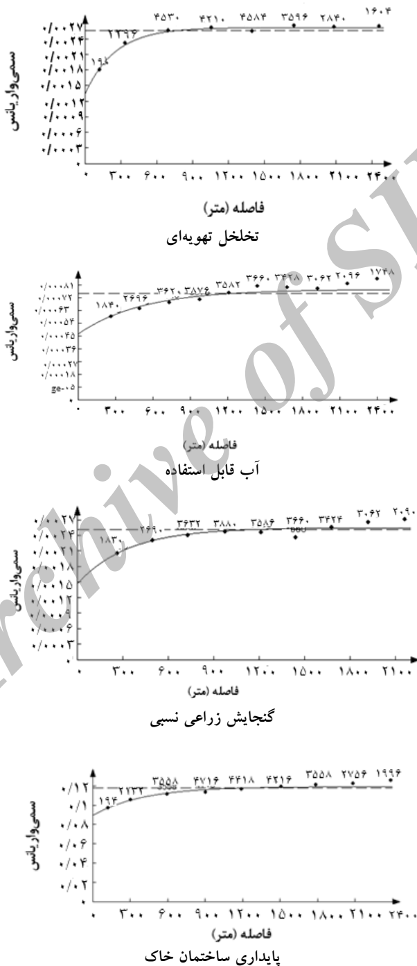
شکل ۳- واریوگرام‌های شاخص‌های فیزیکی کیفیت خاک در عمق صفر تا ۲۰ سانتی‌متر.
