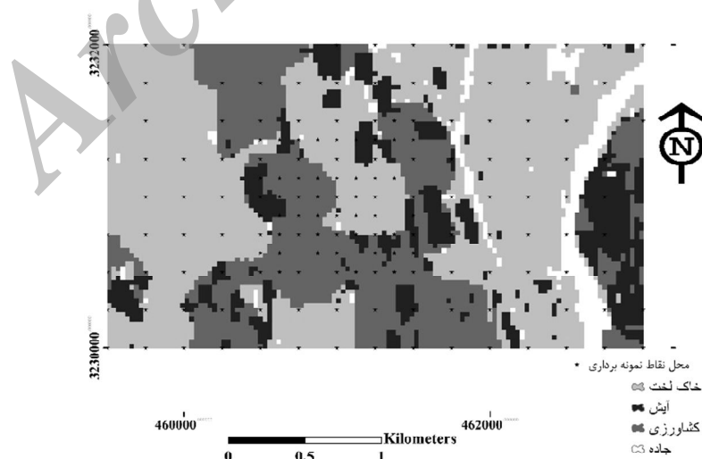
شکل ۴- نقشه کاربری اراضی به همراه موقعیت نقاط نمونه‌برداری.
