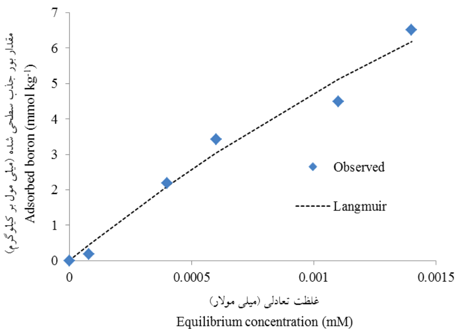
شکل ۴- هم‌دمای جذب سطحی بور و برازش مدل لانگمویر بر داده‌های جذبی کانی بیوتیت.
