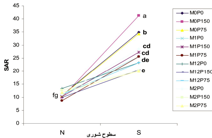
شکل ۲- مقایسه میانگین اثرات متقابل شوری، هیومستر فود و پارس هیومیک بر SAR خاک در شوری ۲ (N) و ۱۰ (S) دسی‌زیمنس بر متر. Figure 2. Comparison of mean interactions of salinity, Humasterfood and Parshumic on SAR in salinity 2 (N) and 10 (S) dS/m.
