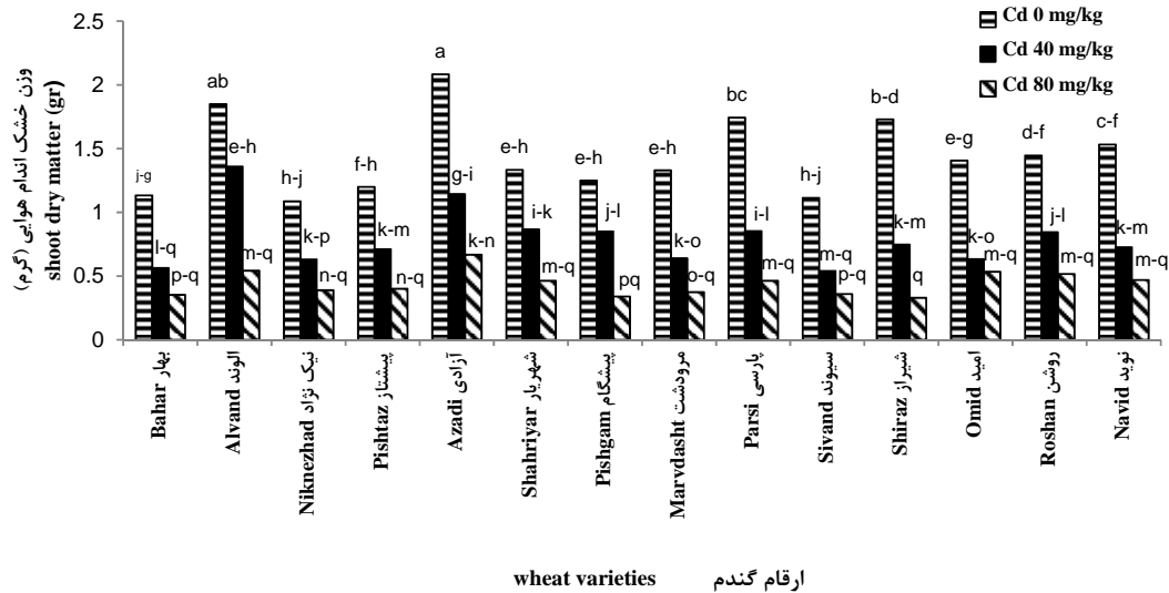
شکل ۳. اثر سطوح مختلف کادمیوم بر وزن خشک بخش هوایی در ارقام مختلف گندم. Fig. 3. Effect of different levels of cadmium on shoot dry weight of different wheat cultivars.
