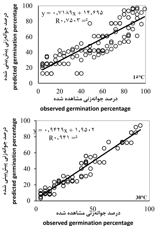
شکل ۲. مقادیر پیش بینی شده درصد جوانه زنی از مدل هیدروتایم در مقابل درصد جوانه زنی مشاهده شده در دماهای مختلف برای بذر Malva sylvestris .
