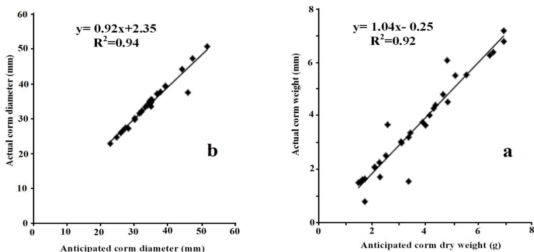
شکل 3- رابطه خطی بین ویژگی‌های پیش‌بینی شده و مشاهده شده بانه زعفران الف) وزن خشک بانه و ب) قطر بانه Fig. 3- Linear relationship between the observed and predicted characteristics of the saffron corm a) corm dry weight, and b) corm diameter
