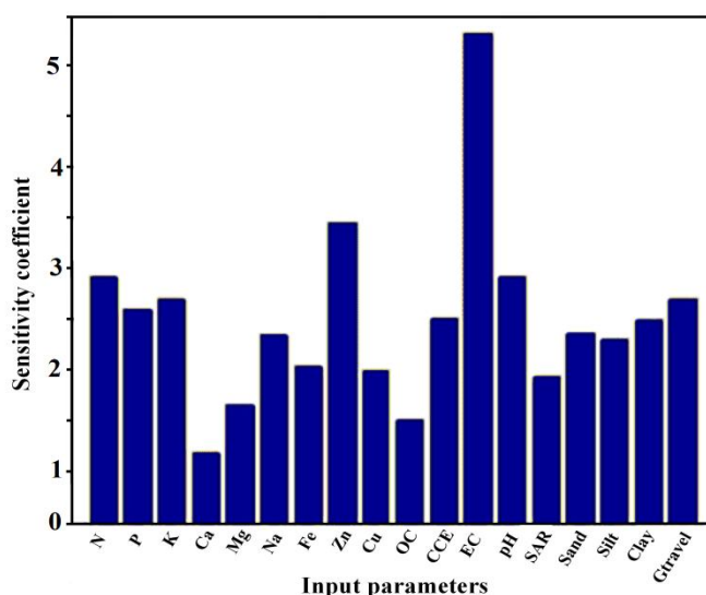
شکل 1- ضرایب حساسیت وزن خشک بانه زعفران
