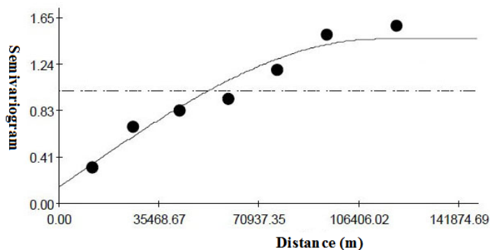
شکل 7- نیم‌تغییرنمای تجربی و مدل برازش داده شده به آن برای بارش بهاره Fig. 7- Experimental semivariogram and the fitted model for spring rainfall
