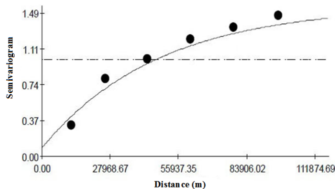
شکل 3- نیم تغییر نمای تجربی و مدل برازش داده شده به آن برای بارش سالانه Fig. 3- Experimental semivariogram and the fitted model for annual rainfall
