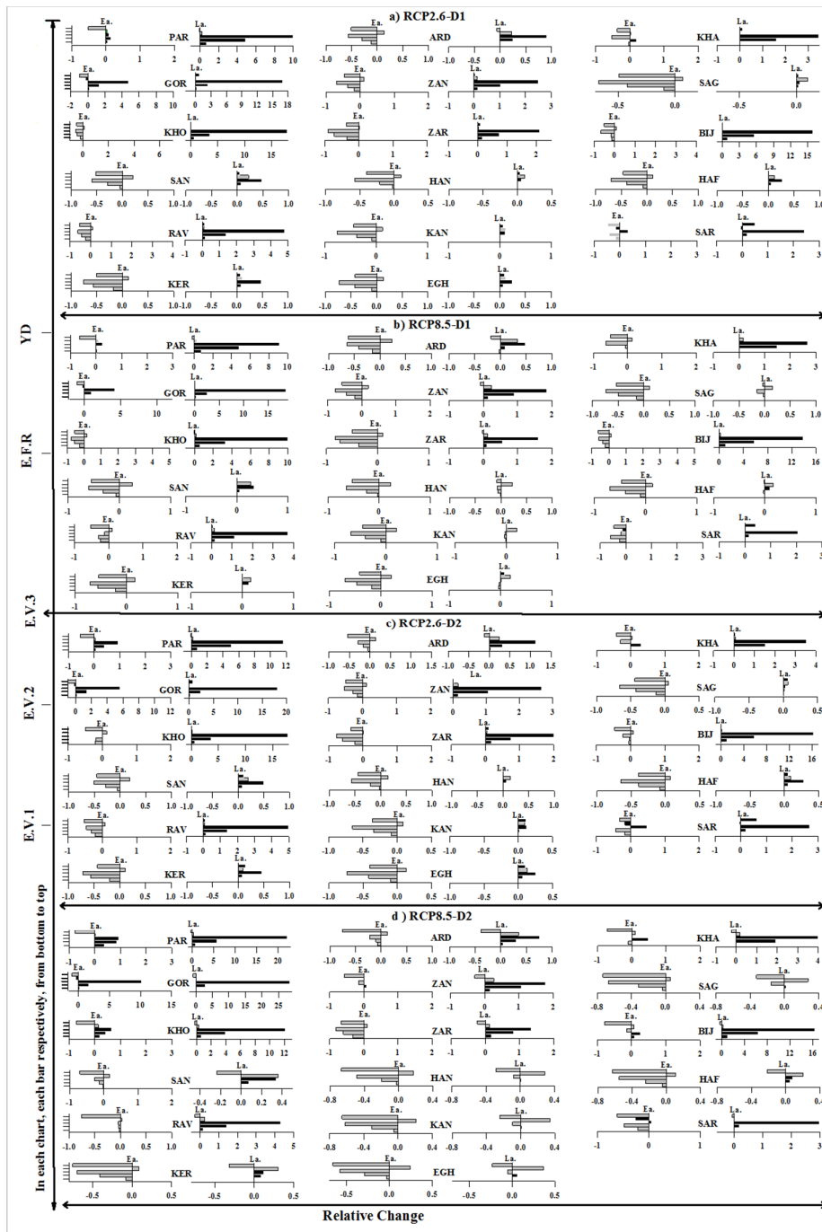
شکل 5- تغییرات نسبی تابش خورشیدی مؤثر (E.F.R)، احتمال وقوع حداقل سه (E.V.3)، دو (E.V.2) و یک (E.V.1) پدیده نامطلوب و YD، برای ارقام زودرس Ea. و دیررس La. در مقایسه با رقم میان‌رس Me. در دوره پایه (1975-2005) برای هر ایستگاه. a) سناریوی RCP2.6 در دوره (2045-2065)، b) سناریوی RCP8.5 در دوره (2045-2065)، c) سناریوی RCP2.6 در دوره (2080-2100) و d) سناریوی RCP8.5 در دوره (2080-2100). رنگ خاکستری و سیاه میله‌ها به ترتیب حاکی از مطلوب‌تر شدن و نامطلوب‌تر شدن شرایط در آینده دارد
