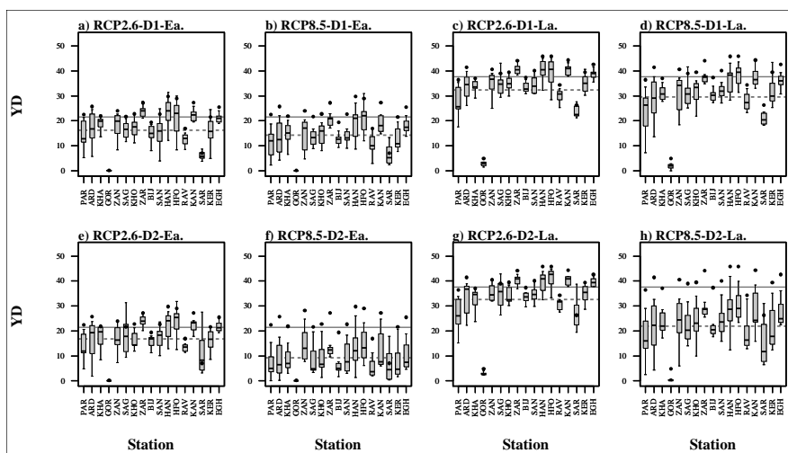
شکل 3- همانند شکل 2 با این تفاوت که برای متوسط کاهش نسبی عملکرد تحت شرایط تنش رطوبتی (YD) در هر فصل رشد
