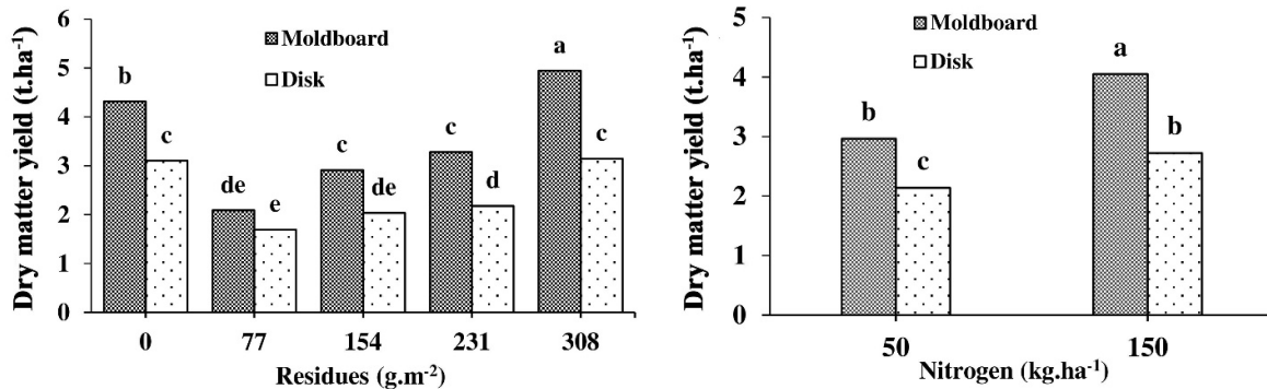
شکل 4- مقایسه‌های میانگین اثر خاک‌ورزی بر عملکرد ماده خشک پنبه رقم خرداد در (a) سطوح مختلف بقایای جو و (b) مقادیر مختلف نیتروژن Fig. 4- Means comparison for the effect of tillage method on dry matter yield of cotton (cv. Khordad) in (a) different levels of plant residues, and (b) different nitrogen levels
