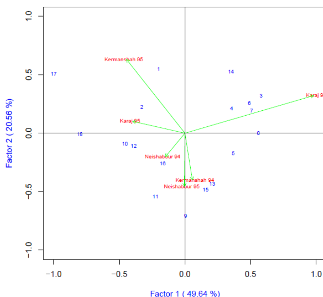
شکل ۲- بای‌پلات حاصل از مقادیر IPCA_1 و IPCA_2 ژنوتیپ‌ها و محیط‌ها Fig. 2- Biplot resulting from IPCA_1 and IPCA_2 values of genotypes and environments
