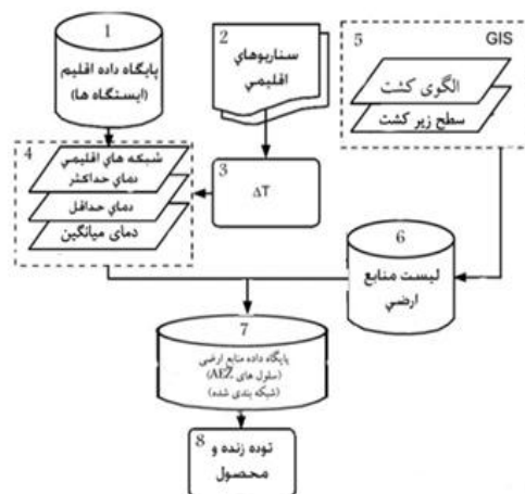
شکل ۲- نمودار جریان‌ی روش AEZ/GIS
