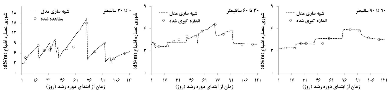
شکل ۴- مقایسه‌ی شوری عصاره اشباع اندازه‌گیری و شبیه‌سازی شده محصول کنجد برای صحت‌سنجی مدل
