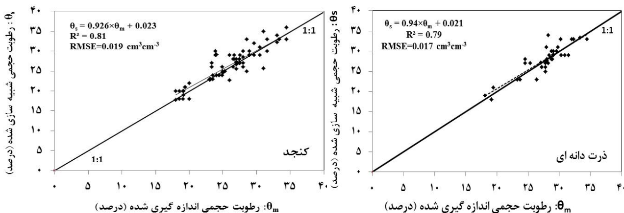
شکل ۳- مقایسه مقادیر رطوبت اندازه‌گیری و شبیه‌سازی شده توسط SWAP برای تمام داده‌های واسنجی و صحت‌سنجی
