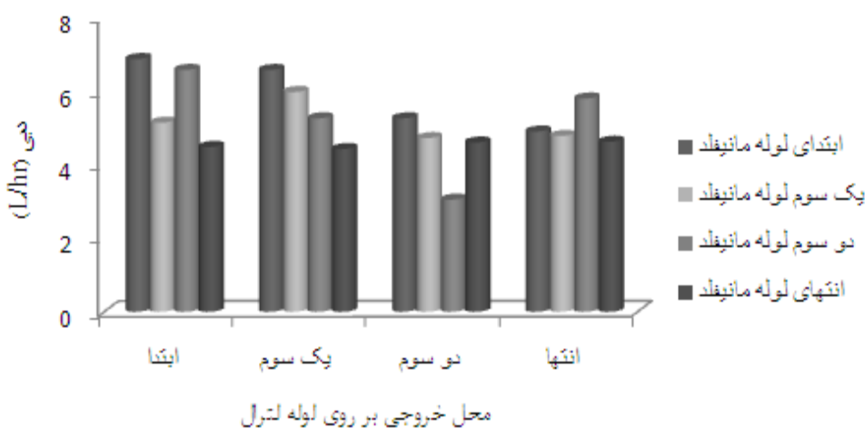
شکل 3- تغییرات دبی قطره‌چکان‌های لوله‌های لترال در مانیفلد آزمایشی مربوط به واحد U_4
