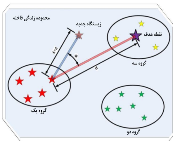
شکل 4- مهاجرت یک فاخته به سمت زیستگاه هدف
