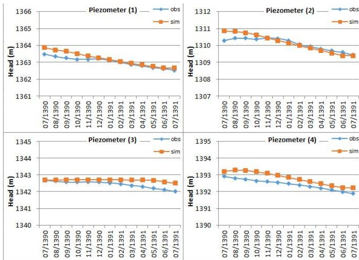
شکل 7- مقادیر سطح ایستایی محاسبه شده و مشاهداتی در انتهای دوره شبیه‌سازی برای چهار پیزومتر منتخب در دوره صحت سنجی
