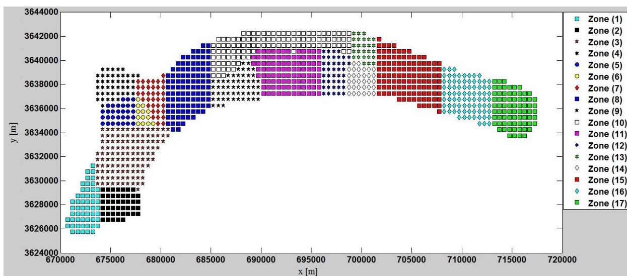
شکل 5- طبقه بندی سطح سفره آب زیرزمینی به 17 منطقه همگن در محیط برنامه‌نویسی MATLAB
