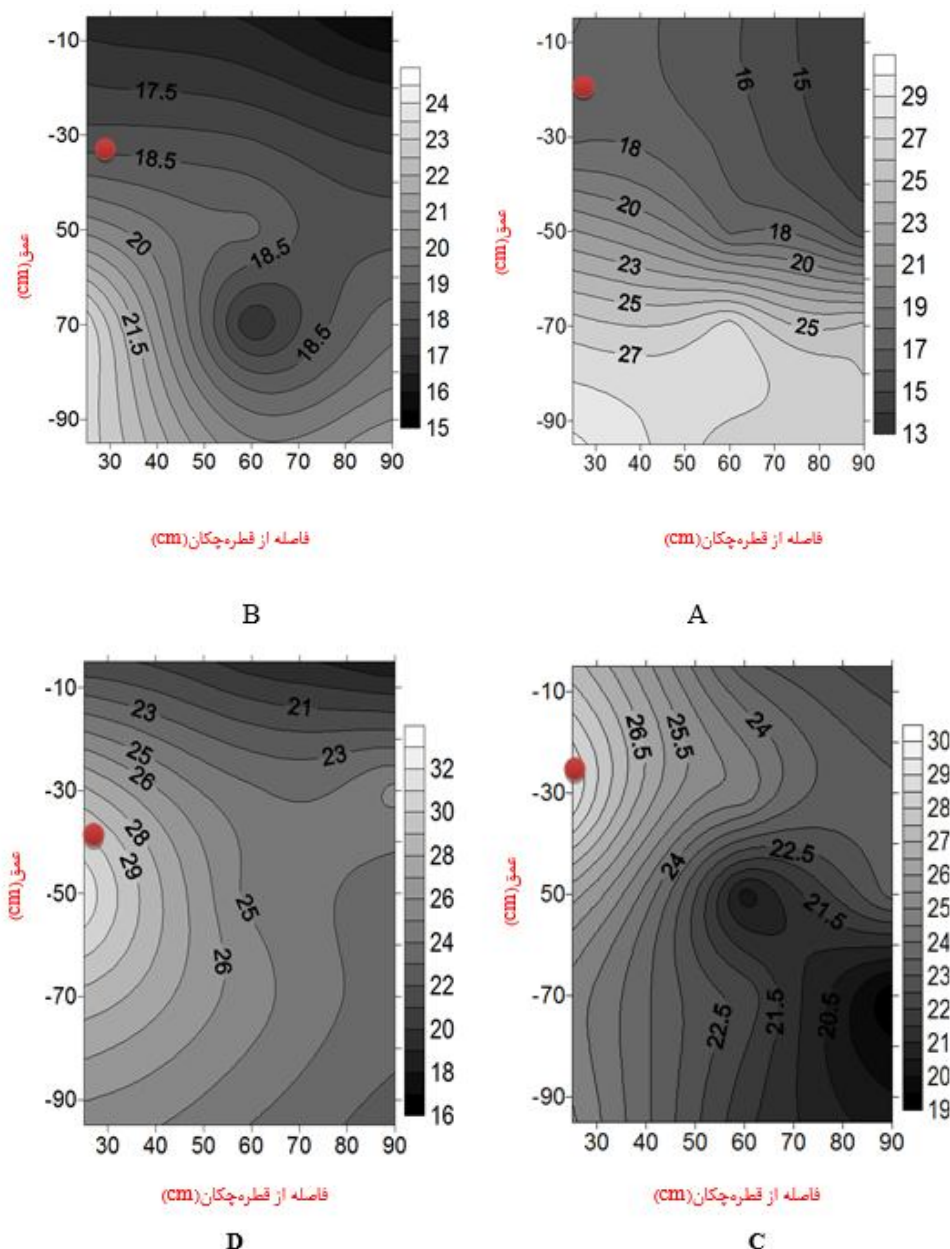
شکل 4- توزیع رطوبت در جهت افقی و عمودی در باغ پرتقال
