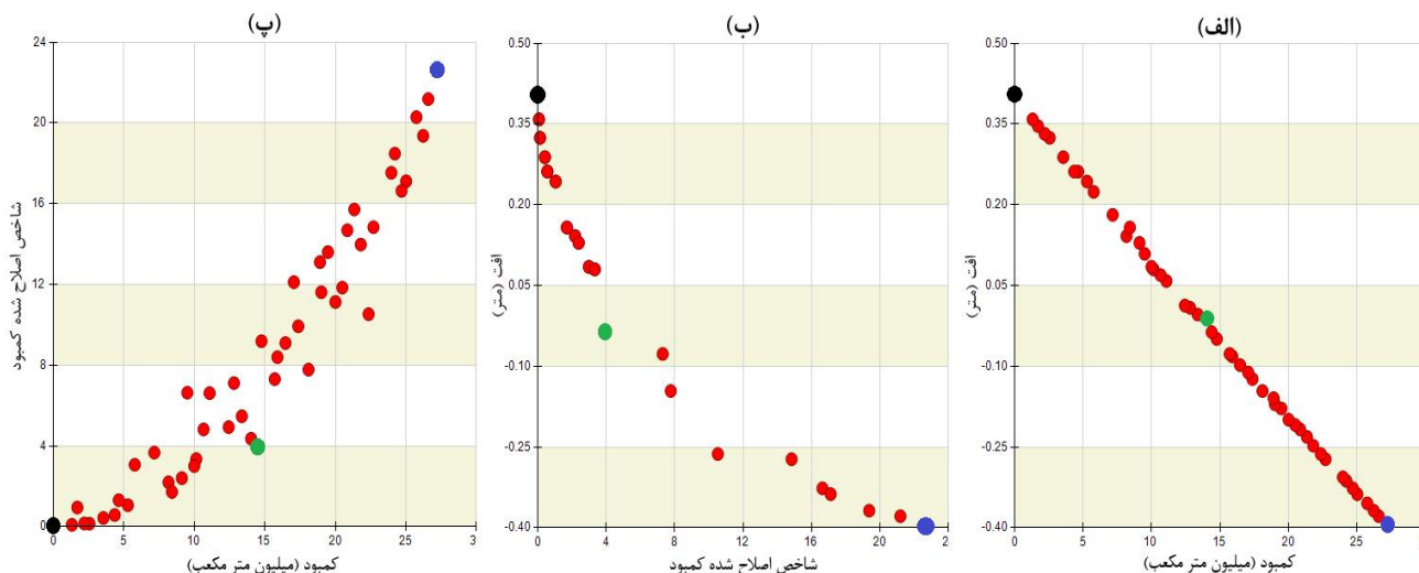
شکل ۵- مقایسه دو به دو جبهه پارتوی اهداف با یکدیگر به صورت دوبعدی
