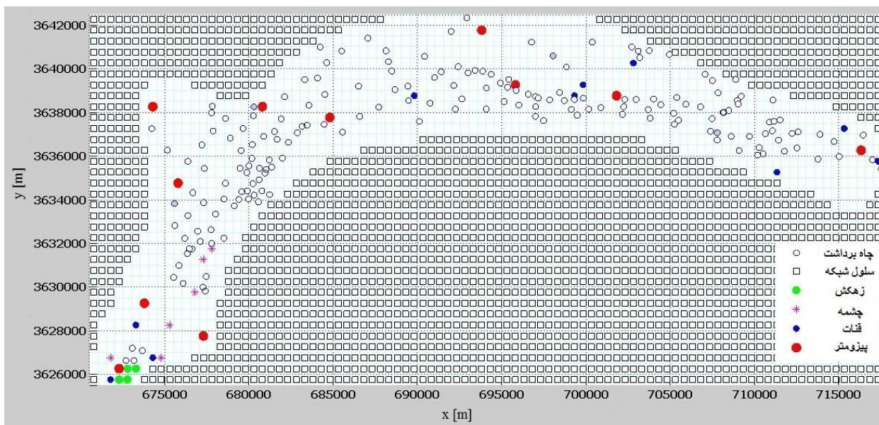
شکل ۳- شبکه بندی آبخوان و موقعیت چاه‌ها، پیزومترها و زهکش منطقه مورد مطالعه در محیط برنامه‌نویسی MATLAB
