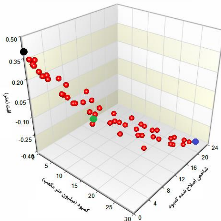
شکل ۴- جبهه پارتو حاصله از مقادیر توابع هدف
