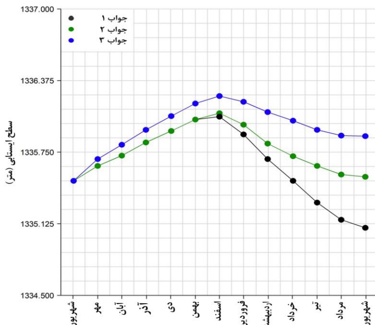
شکل ۷- مقادیر تغییرات سطح ایستابی در طول دوره شبیه‌سازی برای هر یک از سه نمونه جواب مذکور
