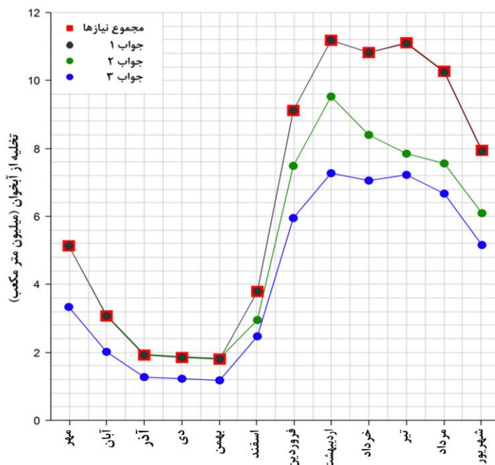
شکل ۶- مجموع مقادیر بهینه برداشت از آبخوان در طول دوره شبیه‌سازی برای سه نمونه از جواب‌های بهینه پارتو
