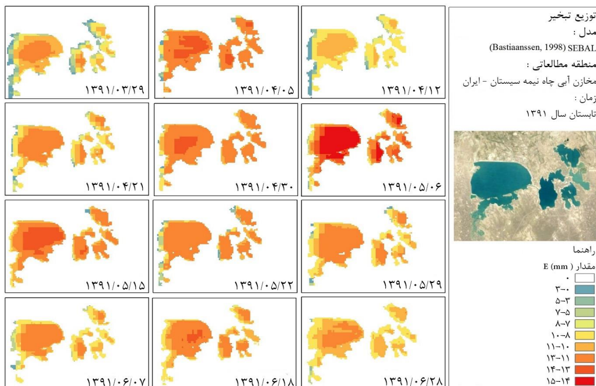
شکل ۷ - مقادیر روزانه تبخیر حاصل از مدل SEBAL
