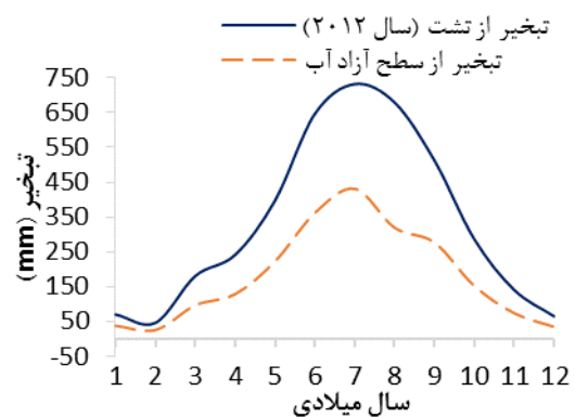
شکل ۲- مقادیر ماهانه تبخیر از تشتک و تبخیر از سطح آب در سال ۲۰۱۲
