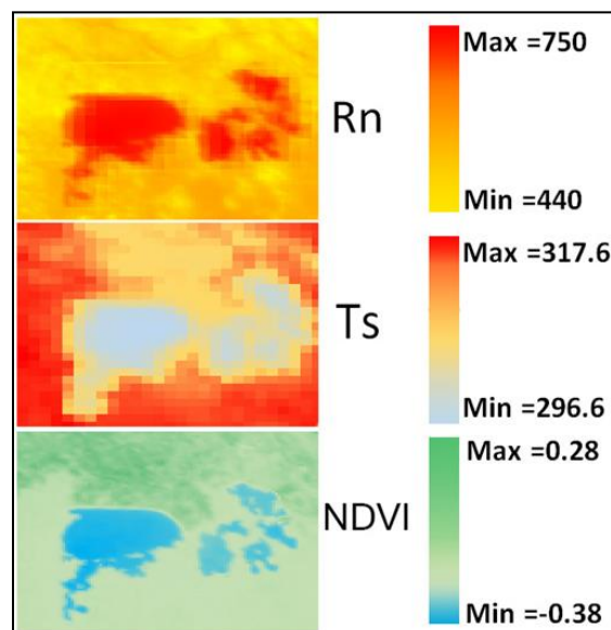
شکل ۴ - توزیع شاخص پوشش گیاهی (NDVI)، دمای سطح زمین (Ts) بر مبنای شار تابش خالص (Rn) برای روز ۳۰ ام تیر ماه ۱۳۹۱، در سطح دشت سیستان با پوشش کامل مخازن چاه نیمه ها و مناطق کشاورزی اطراف.
