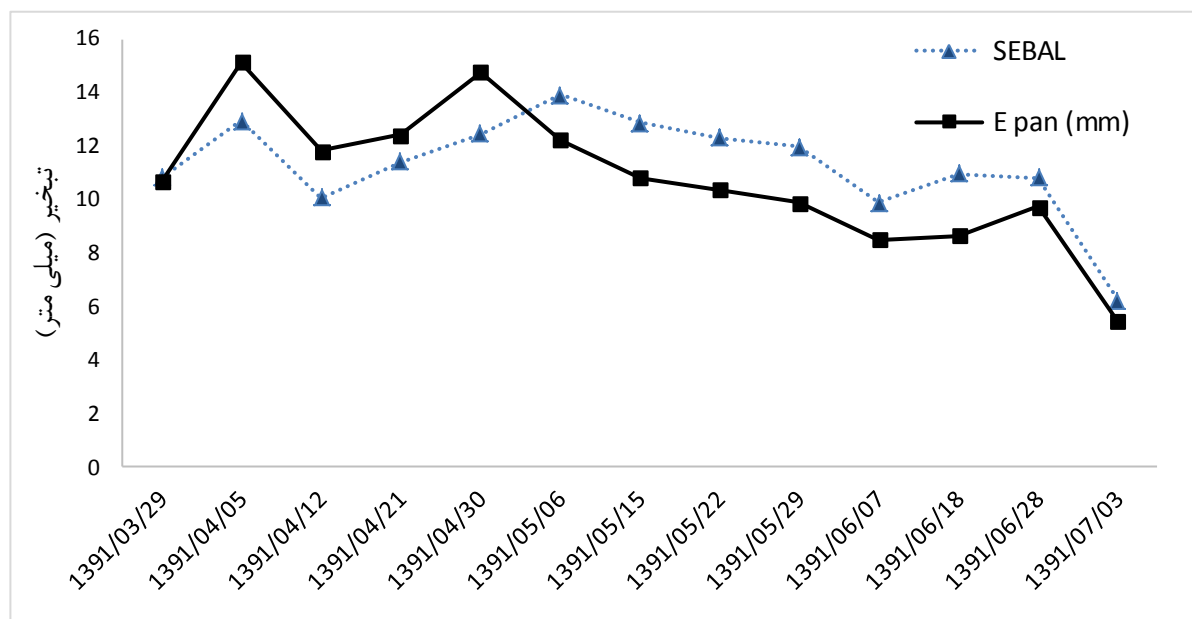
شکل ۸ - روند تغییرات تبخیر روزانه مدل SEBAL در مقایسه با مقادیر روش تشتک (Pan)
