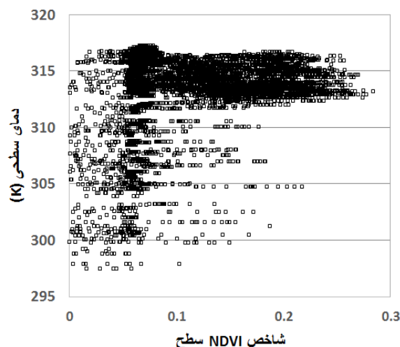
شکل ۵ - توزیع شاخص پوشش گیاهی NDVI، دمای سطح برای
