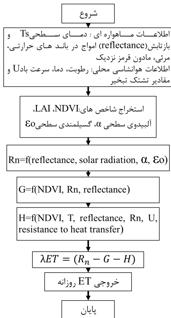
شکل ۳ - فلوجارت محاسبه تبخیر و تعرق روزانه با استفاده از تصاویر ماهواره ای MODIS و مدل SEBAL
