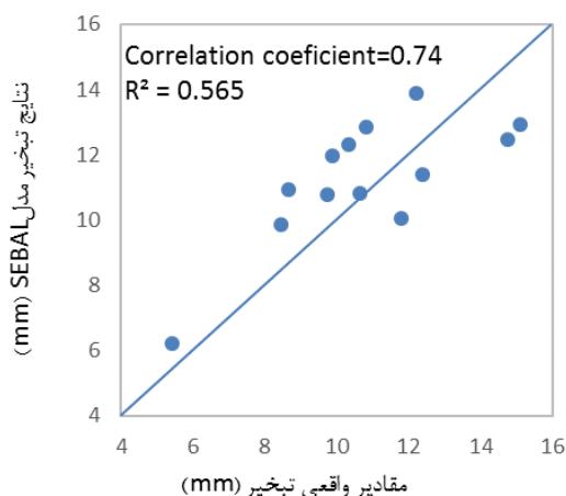
شکل ۶ - مقایسه مقادیر واقعی با مقادیر شبیه سازی شده مدل SEBAL
