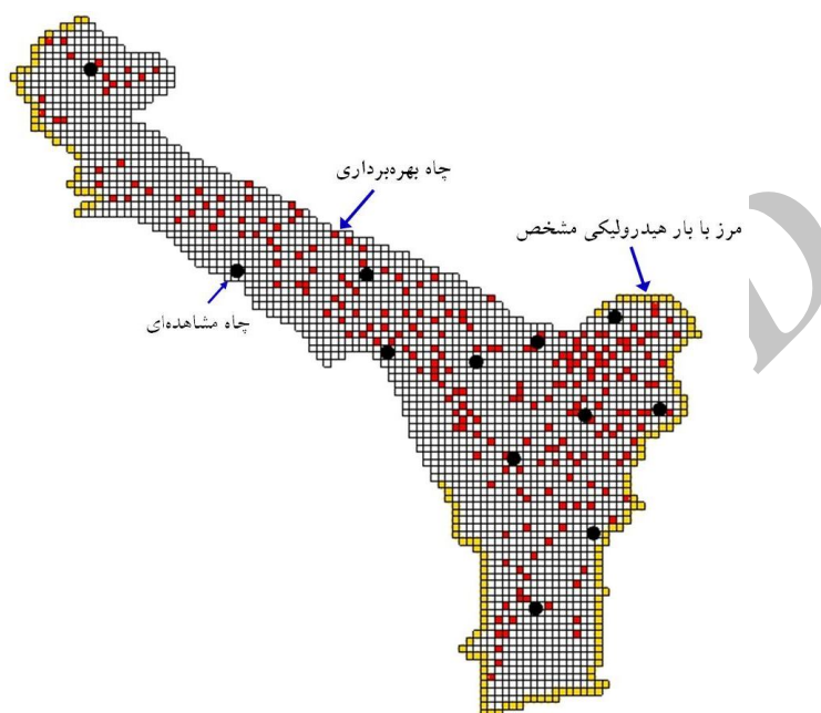
شکل 3- سلول‌های فعال مدل عددی جریان آب زیرزمینی، شرایط مرزی و موقعیت چاه‌های مشاهده‌ای
