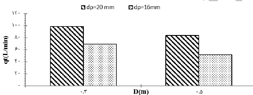
شکل 3- دبی تجمعی برای عمق‌های مختلف کارگذاری در دو قطر مختلف زهکش
