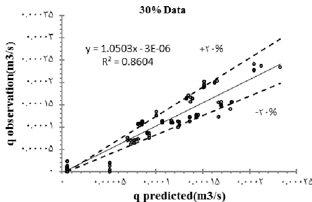
شکل 16- مقایسه نتایج دبی انحرافی در حالت آزمایشگاهی و محاسباتی
