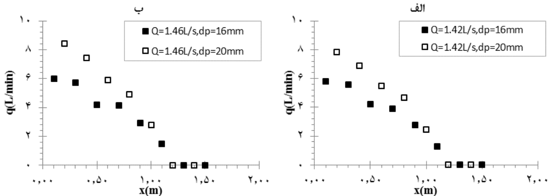
شکل 5- اثر قطر زهکش بر روی دبی زهکش‌ها (الف) شیب 2% (ب) شیب 4%
