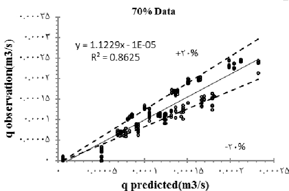
شکل 16- مقایسه نتایج دبی انحرافی در حالت آزمایشگاهی و محاسباتی
