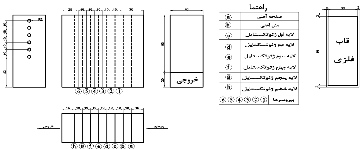
شکل 2- نقشه جعبه فیلتراسیون و قاب‌های استفاده شده (ابعاد به سانتی‌متر است)
