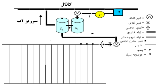
شکل ۱- نمای دستگاه انتقال آب به جویچه‌های آزمایشی
