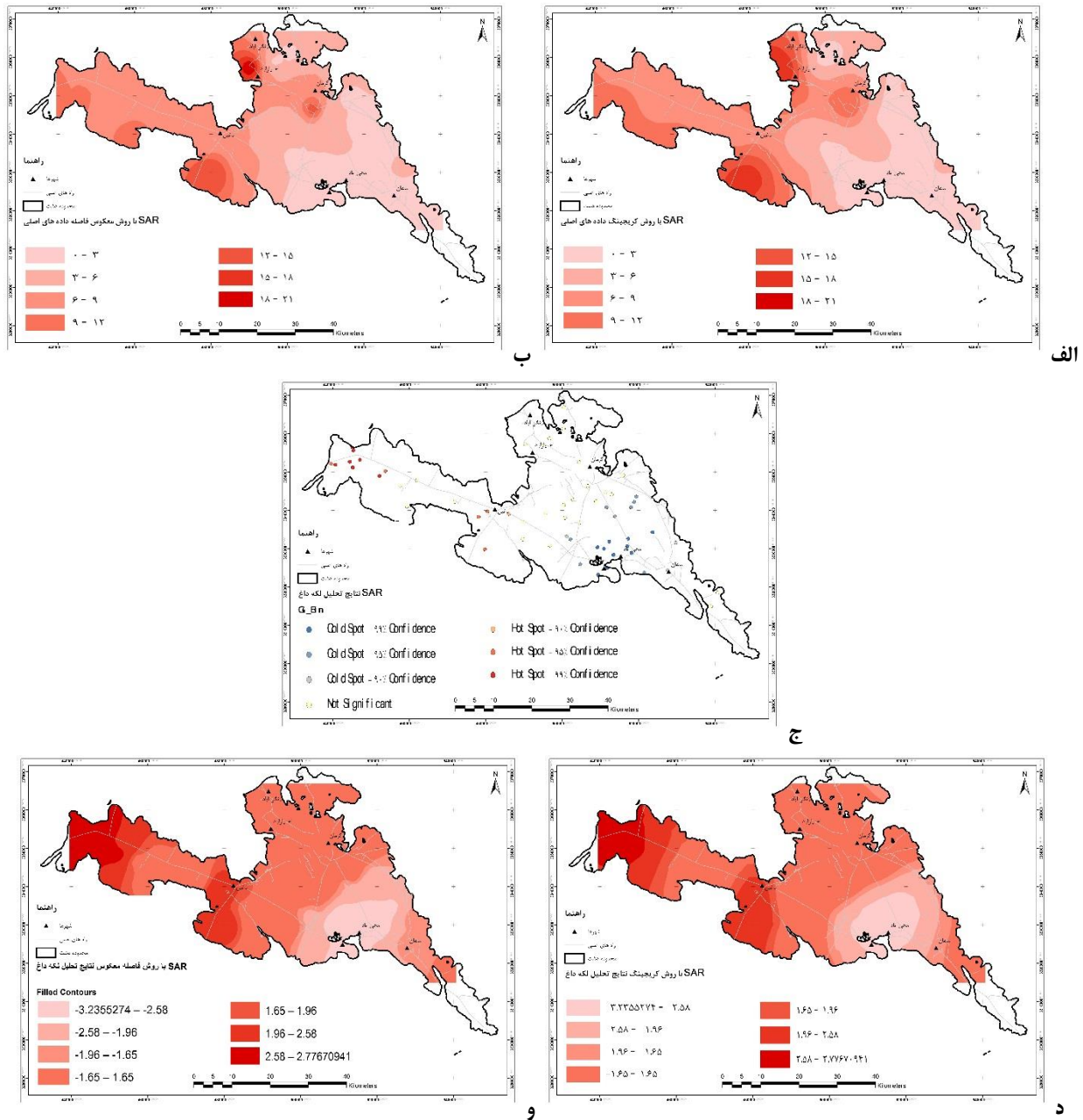
شکل ۵- نقشه های هم مقدار SAR با اعمال روش های: الف) کربجینگ بر روی داده های اولیه، ب) معکوس فاصله وزن دار بر روی داده های اولیه، ج) نتایج تحلیل لکه داغ، د) کربجینگ بر روی نتایج حاصل از تحلیل لکه داغ، و) معکوس فاصله وزن دار بر روی نتایج حاصل از تحلیل لکه داغ.
