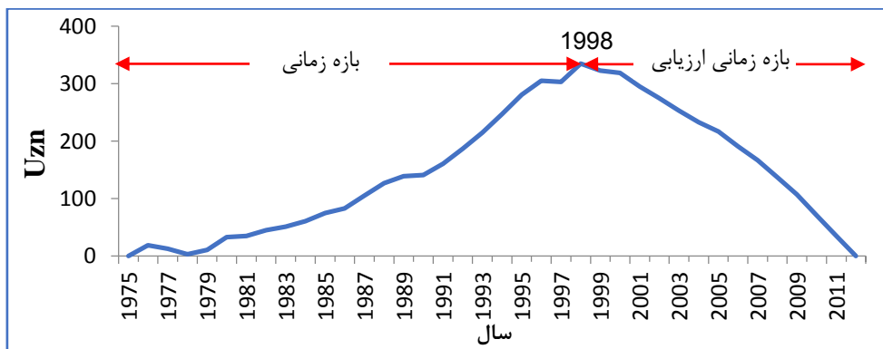
شکل ۴- تغییرات در میانگین سری زمانی دبی سالانه با روش پتیت
