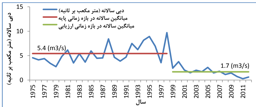
شکل ۵- تغییرات دبی سالانه و میانگین دبی سالانه ایستگاه هیدرومتری ینگ کندی در بازه زمانی پایه و ارزیابی
