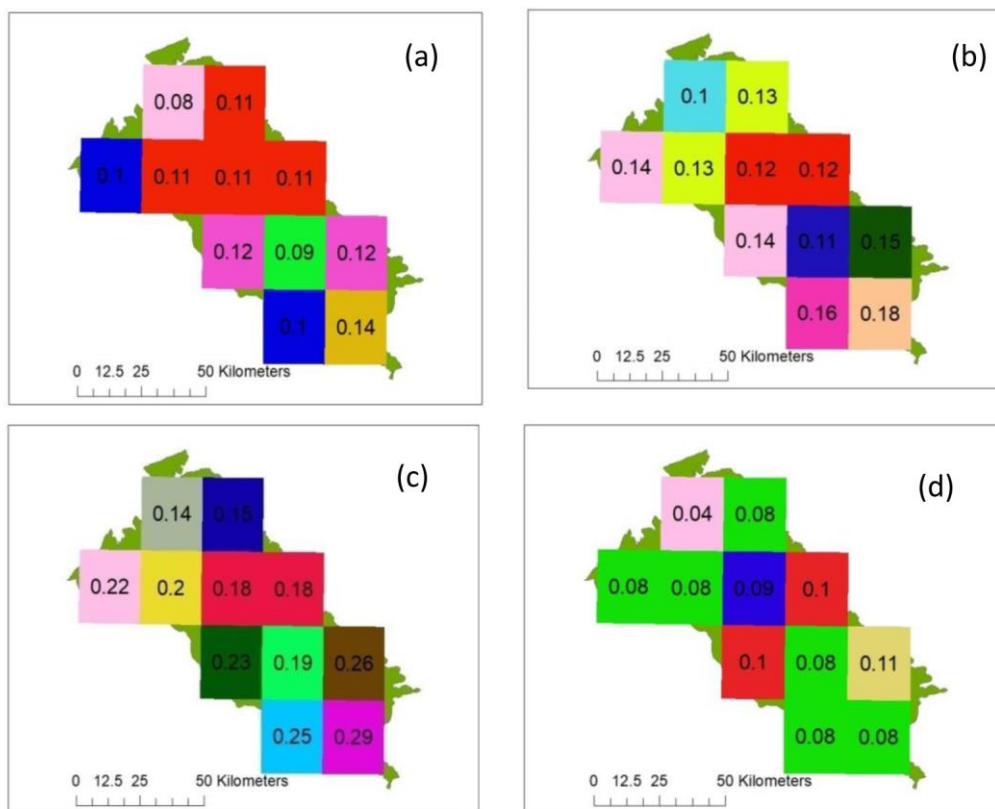
شکل ۲- مقادیر رطوبت خاک (cm 3 /cm 3 ) حاصل از AMSR2 برای روزهای ۹۶/۸/۲۳، (a) ۹۶/۹/۲۷، (b) ۹۶/۱۱/۶، (c) ۹۷/۱/۱۰، (d)
