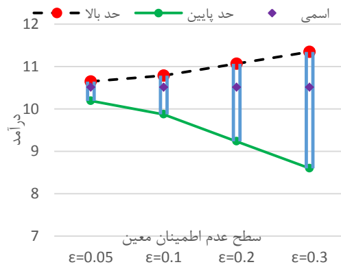
شکل ۴- مقدار اسمی و حد بالا و پایین برای داده خروجی درآمد شبکه آبیاری گتوند در سطوح متفاوت عدم اطمینان
