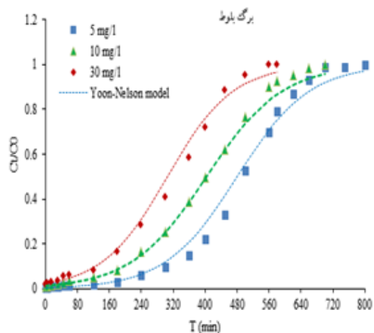
شکل ۸- برازش مدل یون- نلسون بر داده‌های مشاهداتی در غلظت‌های مختلف (ارتفاع بستر ۴۰ سانتی‌متر و دبی ۵۰ میلی‌لیتر در دقیقه)
