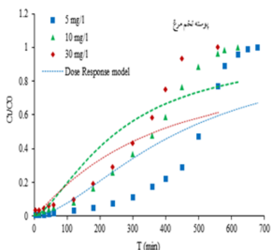
شکل ۹- برازش مدل پاسخ دوز بر داده‌های مشاهداتی در غلظت‌های مختلف (ارتفاع بستر ۴۰ سانتی‌متر و دبی ۵۰ میلی‌لیتر در دقیقه)
