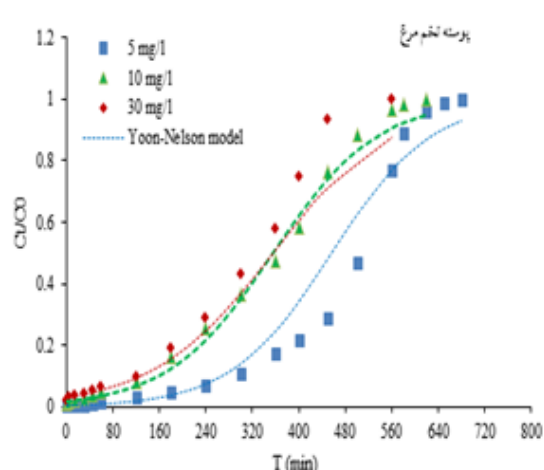
شکل ۸- برازش مدل یون- نلسون بر داده‌های مشاهداتی در غلظت‌های مختلف (ارتفاع بستر ۴۰ سانتی‌متر و دبی ۵۰ میلی‌لیتر در دقیقه)
