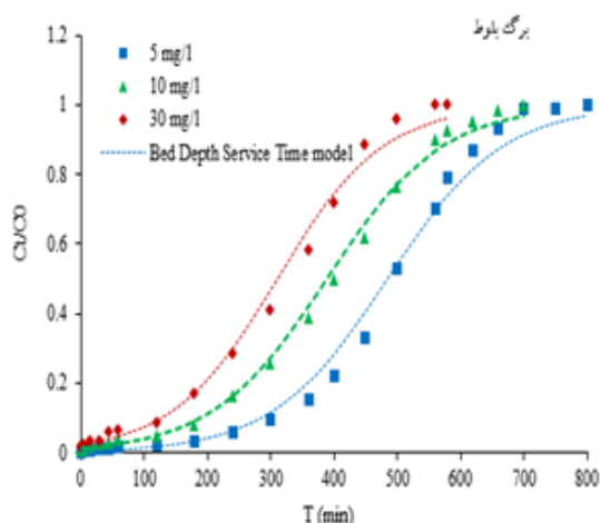
شکل ۱۰- برازش مدل عمق بستر- زمان سرویس بر داده‌های مشاهداتی در غلظت‌های مختلف (ارتفاع بستر ۴۰ سانتی‌متر و دبی ۵۰ میلی‌لیتر در دقیقه)
